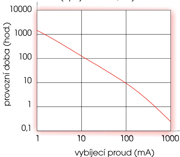
Trvalý vybití proud (vybiteno do 0,9 V)
